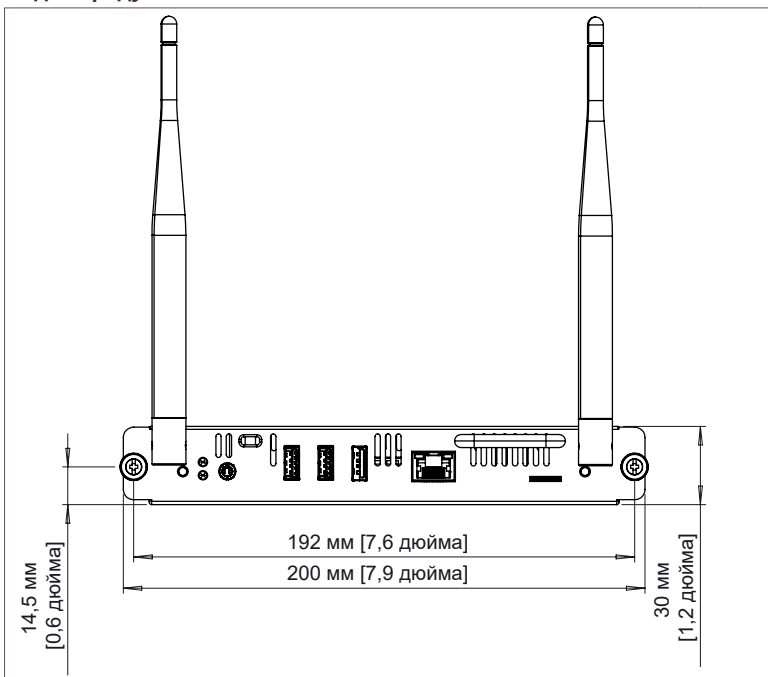
Вид спереду
