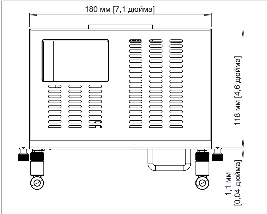
Вид зверху
